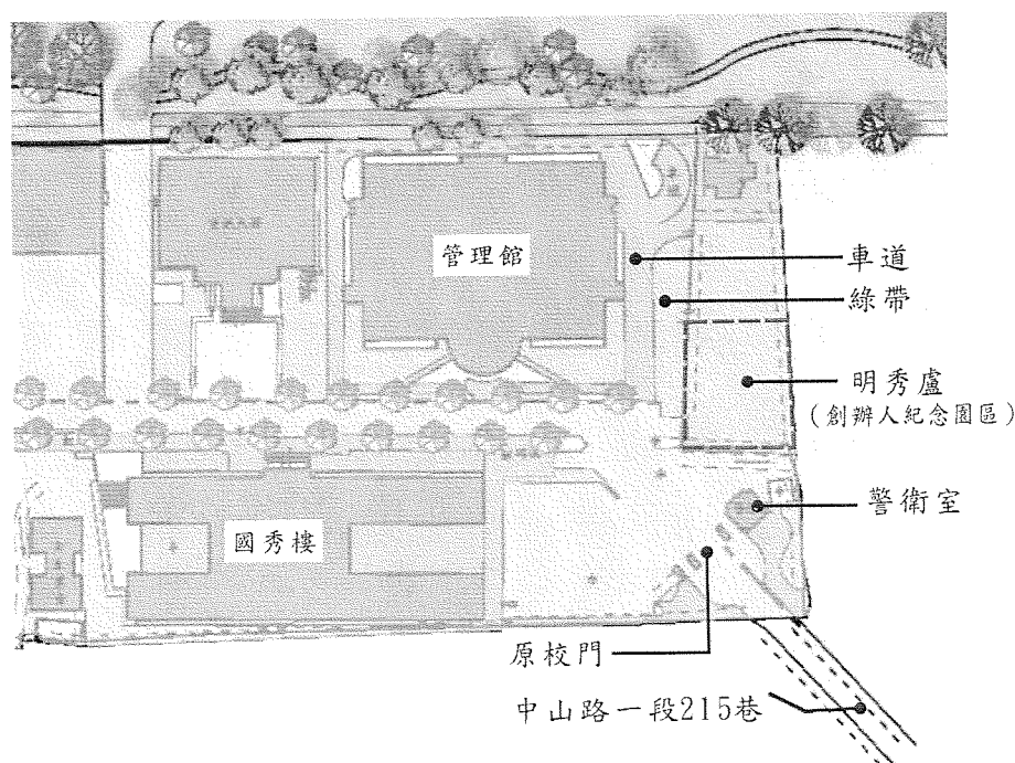
圖 1 基地位置示意圖
